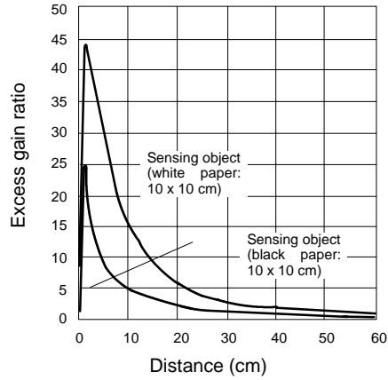
E3F2-DS30□4 E3F2-DS30□4-P1
