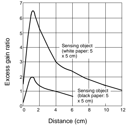
E3F2-DS10Z□
